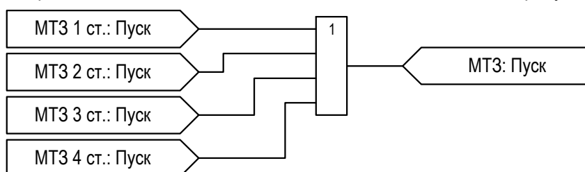
Рисунок 2.22 – Функциональная схема внешней логики МТЗ
